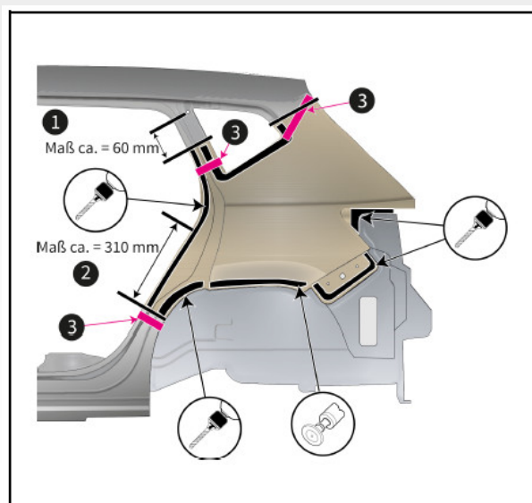
Bild 1: Seitenteil Ausbau
