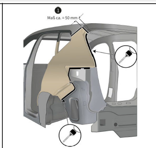
Bild 2: Seitenteil Ausbau, Heckansicht
